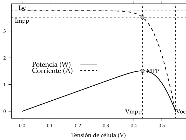
FIGURA 4.6: Curvas corriente-tensión (línea discontinua) y potencia-tensión (línea continua) de una célula solar ( T_a = 20^\circ\text{C} y G = 800 \frac{\text{W}}{\text{m}^2} ).
