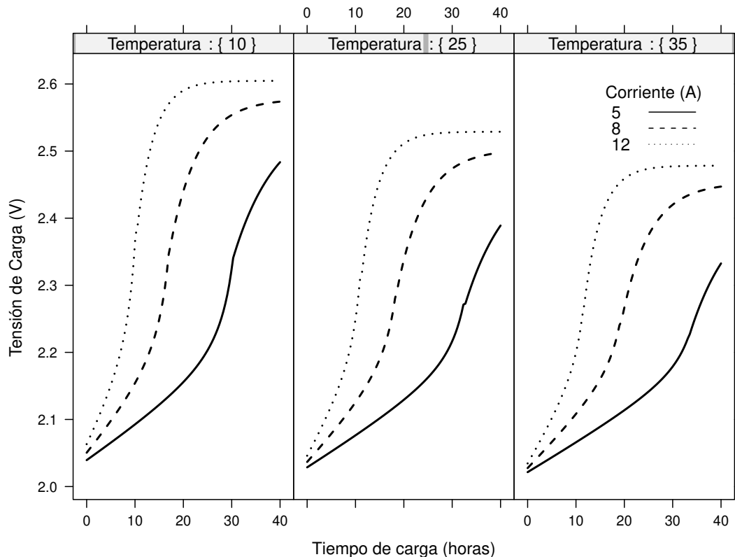
FIGURA 7.3: Curvas de evolución de la tensión en bornes de una batería durante un proceso de carga a corriente constante, para diferentes valores de corriente de carga y temperatura ambiente. Las curvas están particularizadas para una batería con una capacidad C_{10} = 300 Ah. Se ha utilizado el modelo de comportamiento propuesto en la referencia [CLC93].
