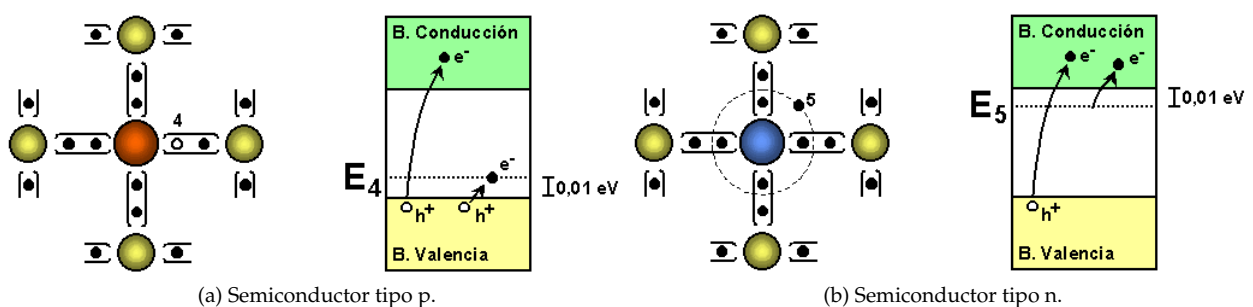
FIGURA 4.1: Semiconductores dopados.
