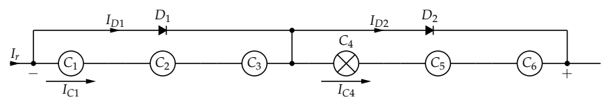
FIGURA 5.4: Colocación de diodo de paso para evitar el fenómeno de punto caliente.
